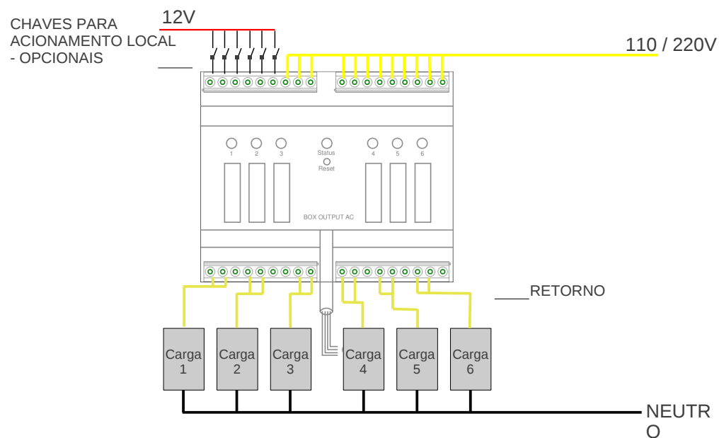
Figura 04 – Instalação padrão.
