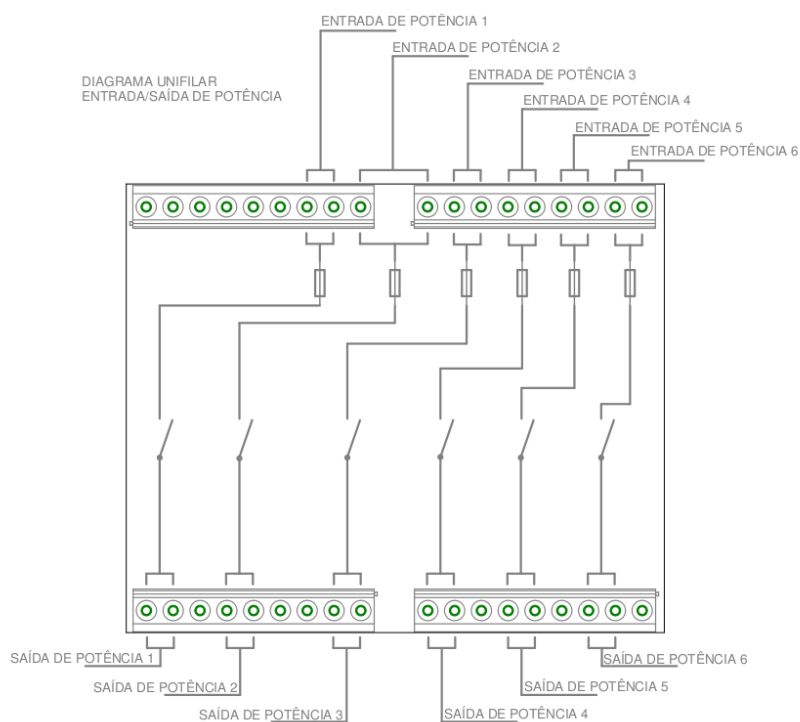
Figura 03 – Diagrama circuito de potência.
